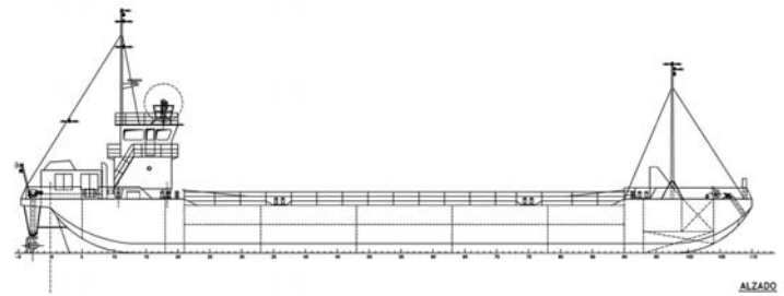
ALZADO
